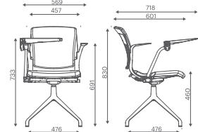
Myko Base Swivel Glide 4-M8PL-M013-M054-M402-A
